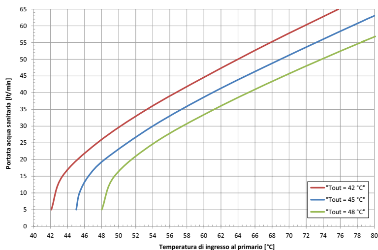
Produzione in continuo ACS (H2FAST-120, Tin 10 °C)
