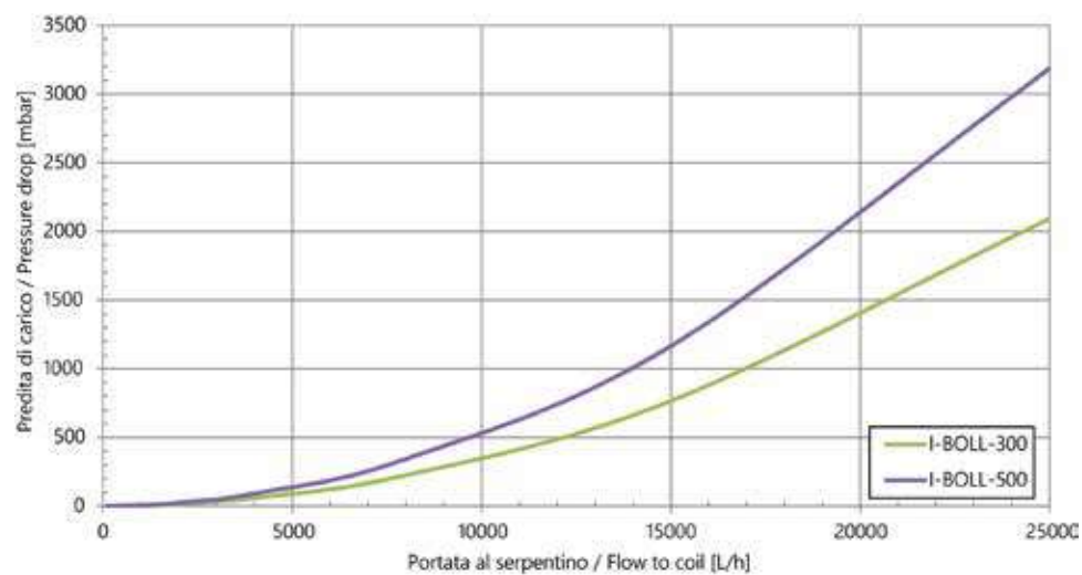
Perdita di carico al serpentino
