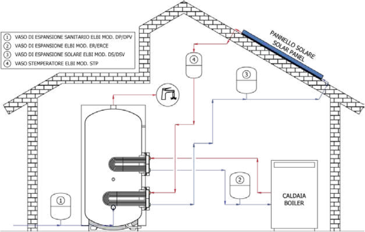
Schema illustrativo; per la realizzazione degli impianti fare sempre riferimento a tecnico abilitato.
