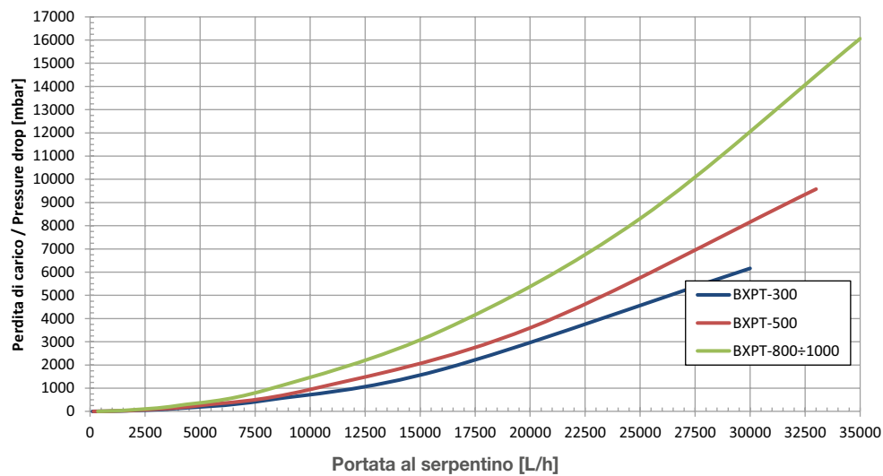
Perdite di carico sul serp. integr.
