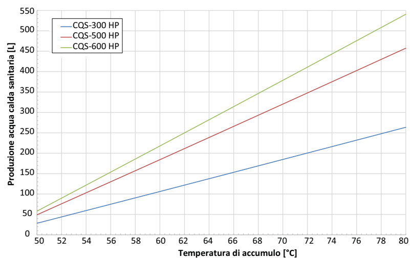
CQP PDC - Produzione teorica acqua sanitaria (ingresso 10 °C, uscita 45 °C)
