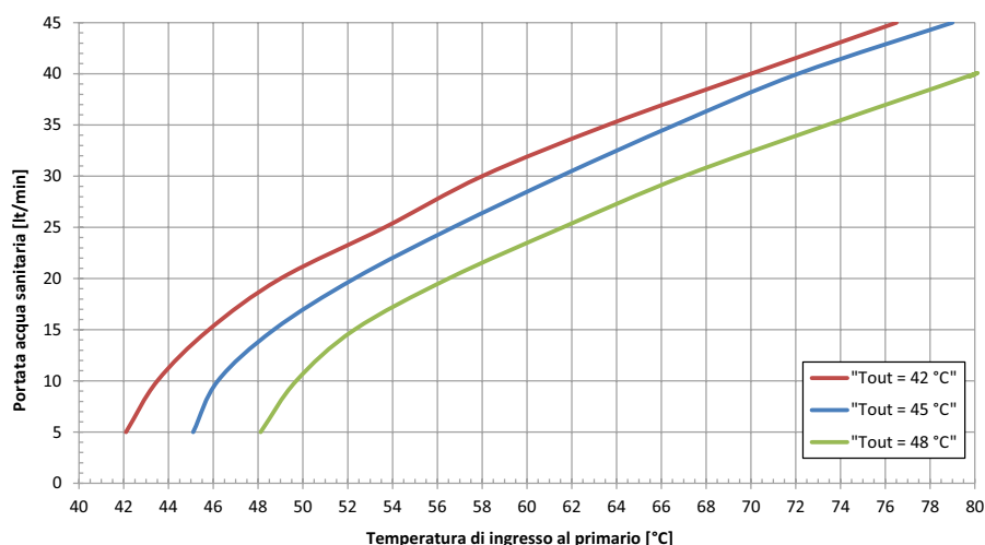
Produzione in continuo ACS (H2FAST-70, Tin 10 °C)
