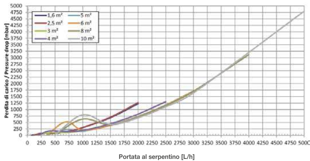
Perdita di carico al serpentino Funzionamento a vapore saturo
