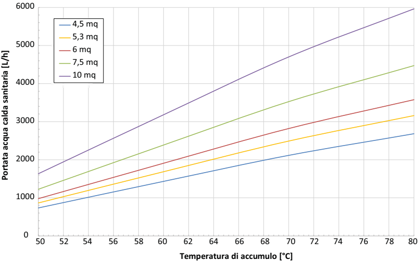
Produzione in continuo acqua sanitaria (ingresso 10 °C, uscita 45 °C)
