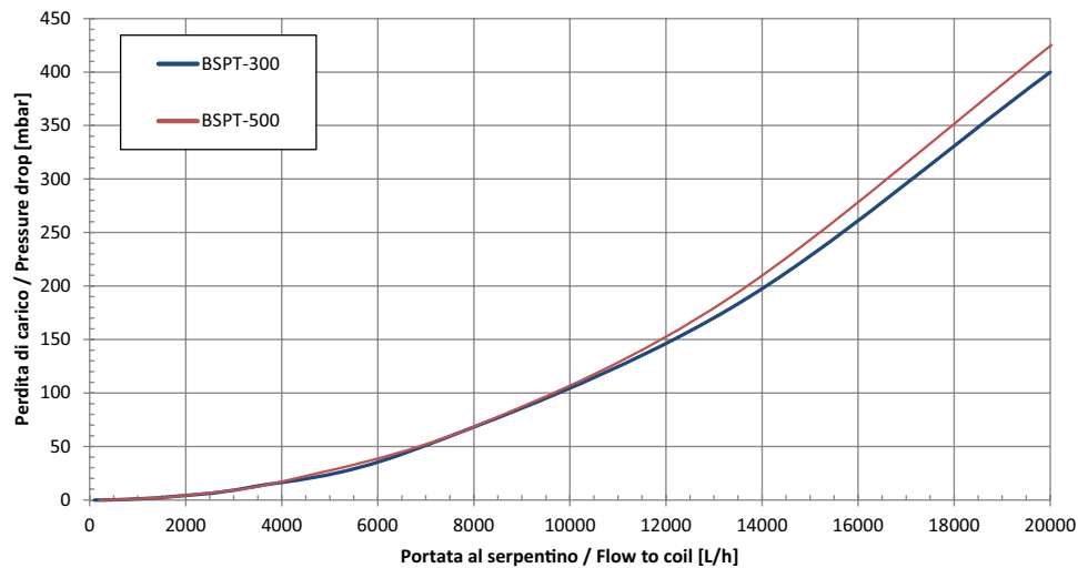
Perdite di carico sul serp. integr. H-BSPT
