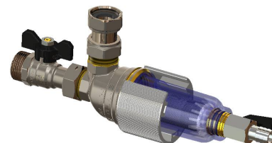
ingresso caldaia boiler inlet
